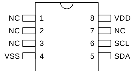
图 2-1 SQ7101 SOP8 封装型态引脚配置
