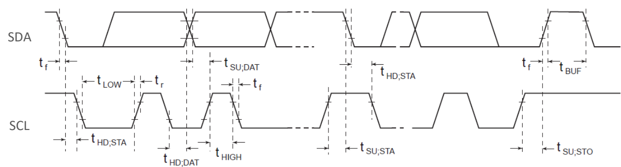
图 3-2 I2C 时序图
