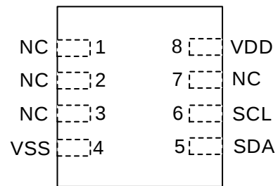
图 2-2 SQ7101 8-Lead DFN 封装型态引脚配置
