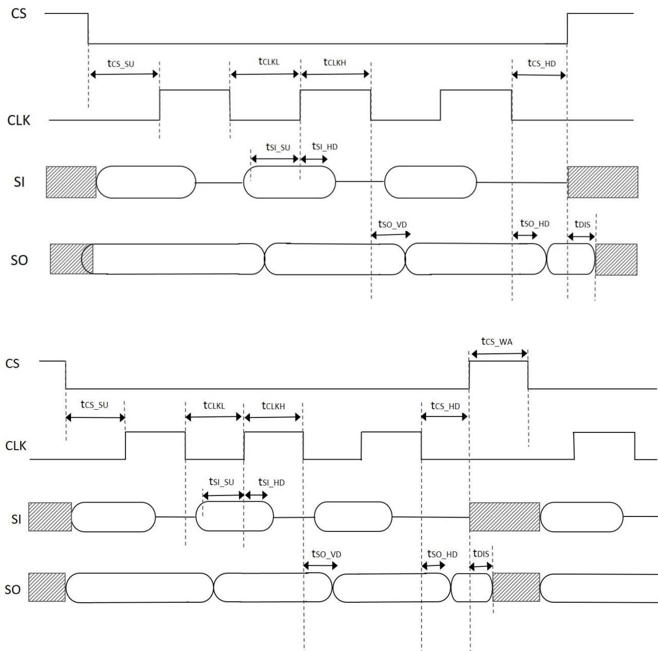
图 3-3 SPI 时序图
